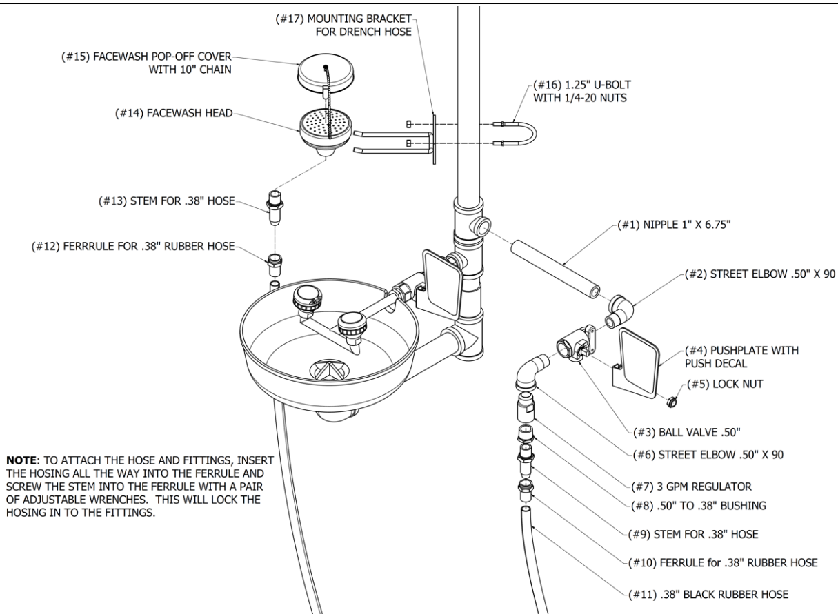
FIGURA #7 ACOPAMIENTO DE LA MANGUERA PARA LAVADO, VÁLVULA Y PLACA DE EMPUJE
