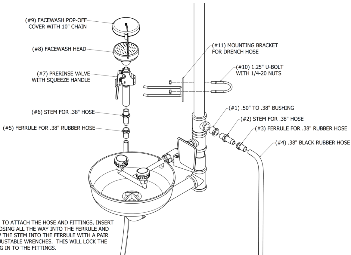
FIGURA #6 ACOPAMIENTO DE LA MANGUERA PARA LAVADO, VÁLVULA Y MANIJA CONTRÁCTIL
